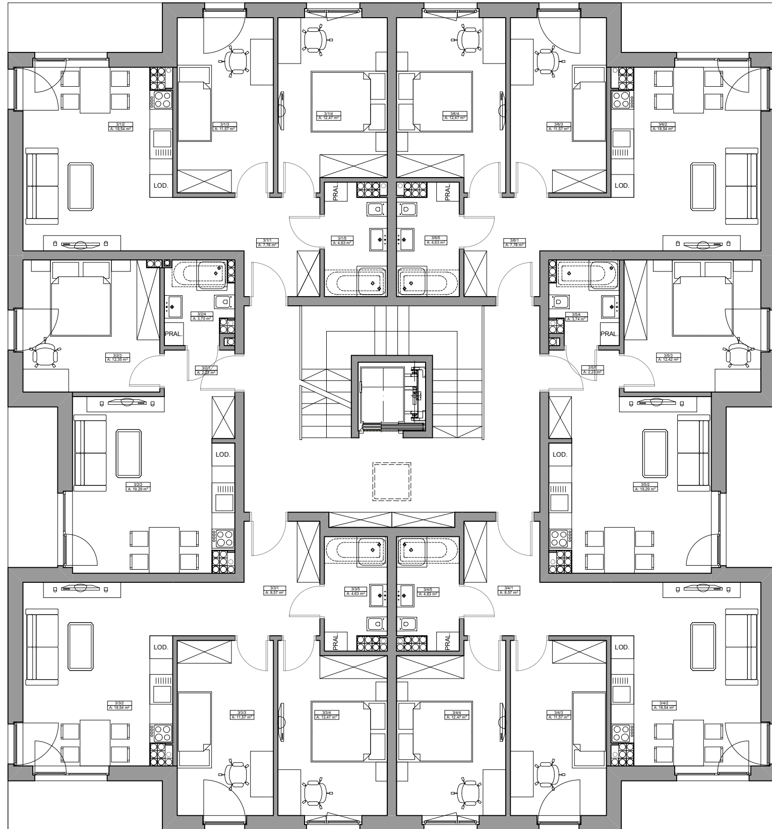
RZUT 3 PIĘTRA
